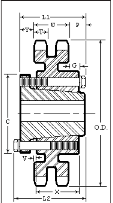
TYPE D120QD_C5
