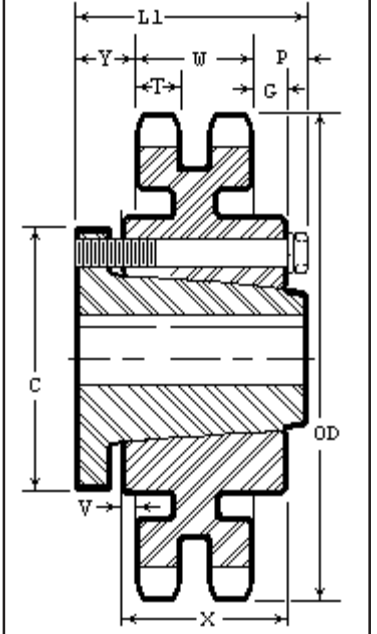
TYPE D120QD_C6
