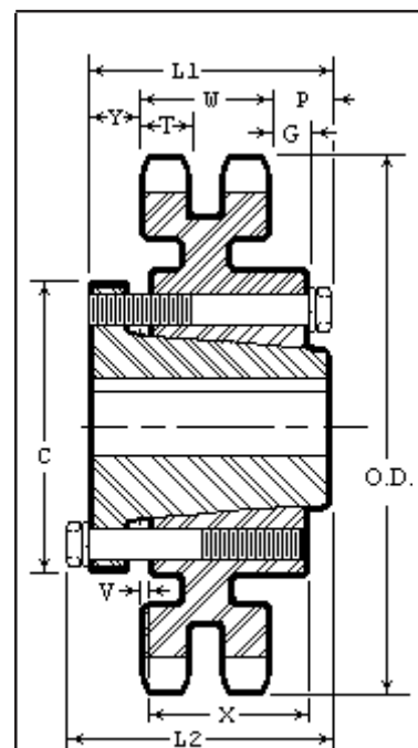
TYPE D140QD_C5
